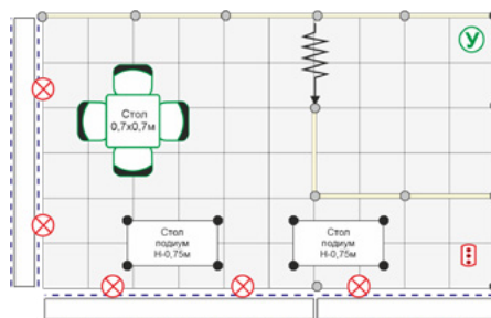
СХЕМА СТЕНДА (УГЛОВОЙ)
